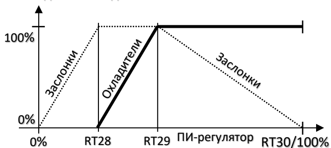
Охлаждение: охладитель и заслонки
