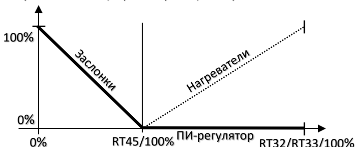
Нагрев: заслонки (первая ступень) и нагреватели
