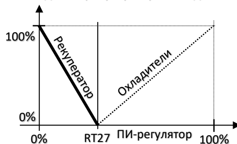
Охлаждение: рекуператор и охладители
