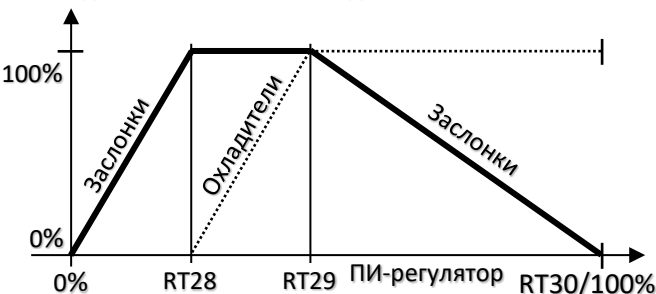
Охлаждение: заслонки и охладители
