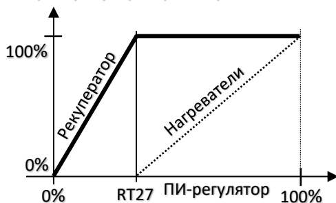
Нагрев: рекуператор и нагреватели
