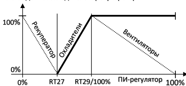
Охлаждение: охладитель и рекуператор
